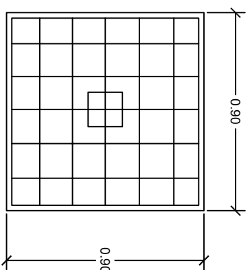
แผ่นขยายฐานราก F1
