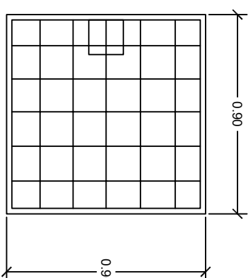
แผ่นขยายฐานราก F2
